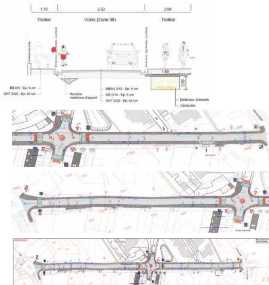
COUPE CC' (Chemin de Trinchet)
